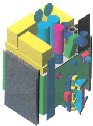
Astrosat
