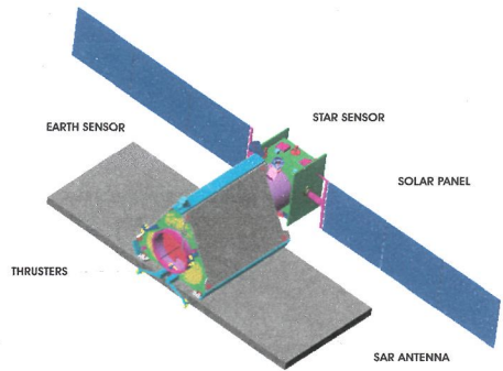
RISAT
